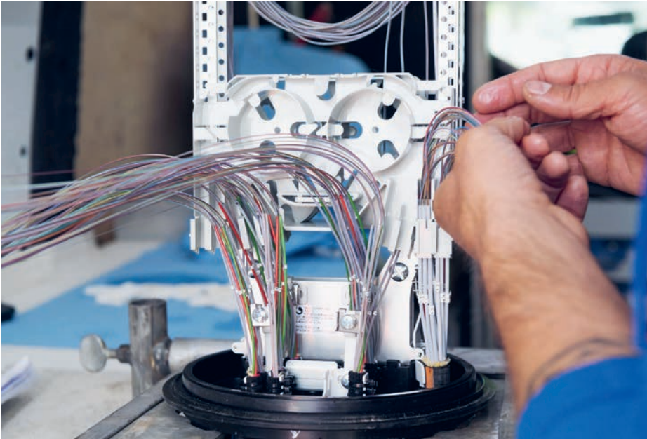
Einbau Glasfaser
